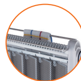
RADIADOR MICATHERMIC JATA 1.200/2.000W. Termostato regulable. Dispositivo de seguridad antivuelco y protección contra sobrecalentamiento. Barras superiores abatibles. 64x75,5x13cm.
